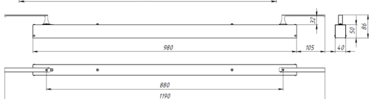
Рисунок 4 - Габаритные размеры при комплектации с креплением для реечного потолка на примере Line 980мм.
